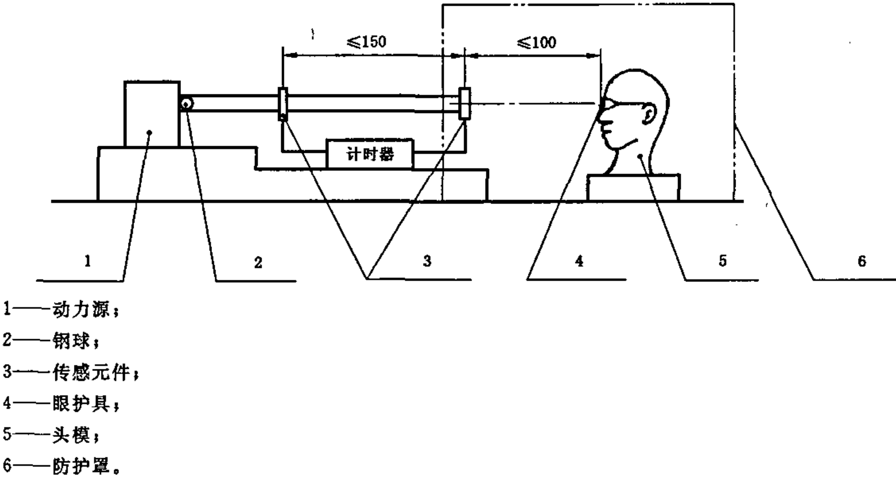
图 4 抗高速粒子冲击试验装置
