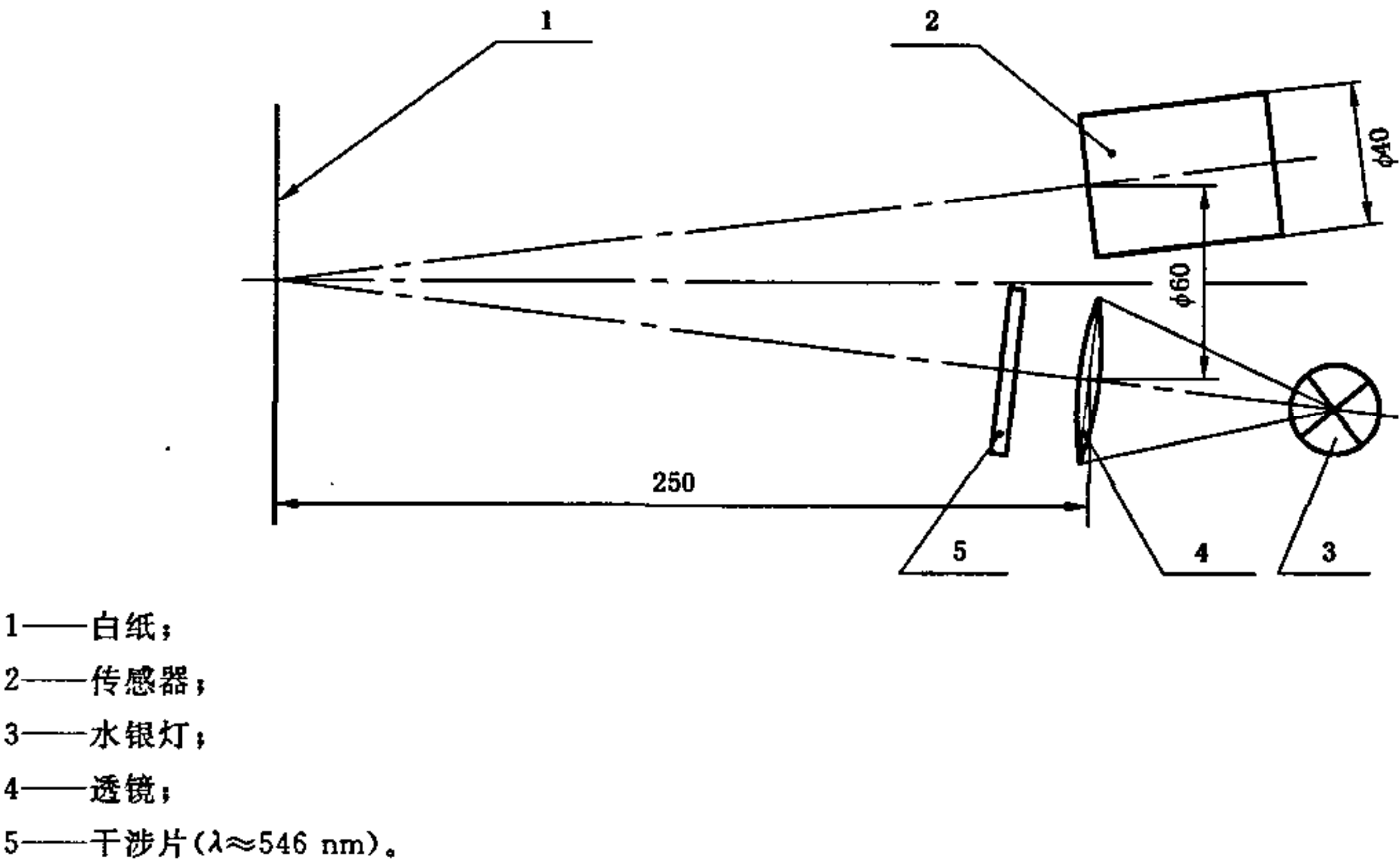
图 9 光电反射计
